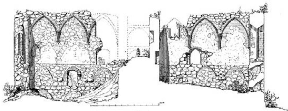
Abb. 24. Papau. – Schnitt durch Capelle und Capelsaal. A–B Abb. 25.
